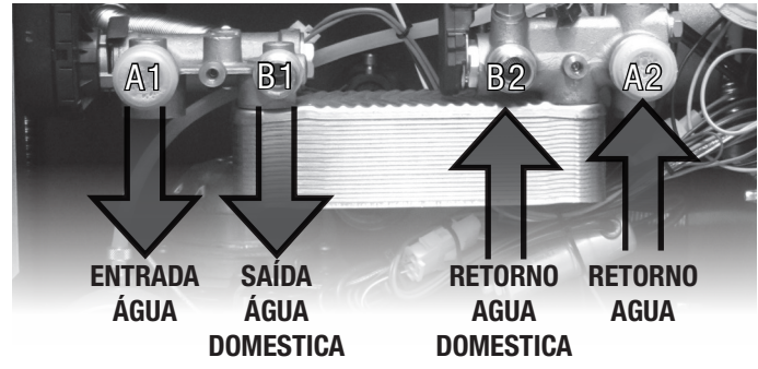
Diagrama de ligação para termo estufa com kit de água quente sanitária
