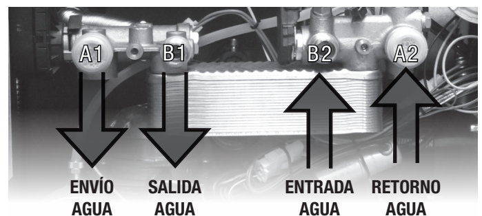
Esquema conexión estufa con kit de producción de agua sanitaria
