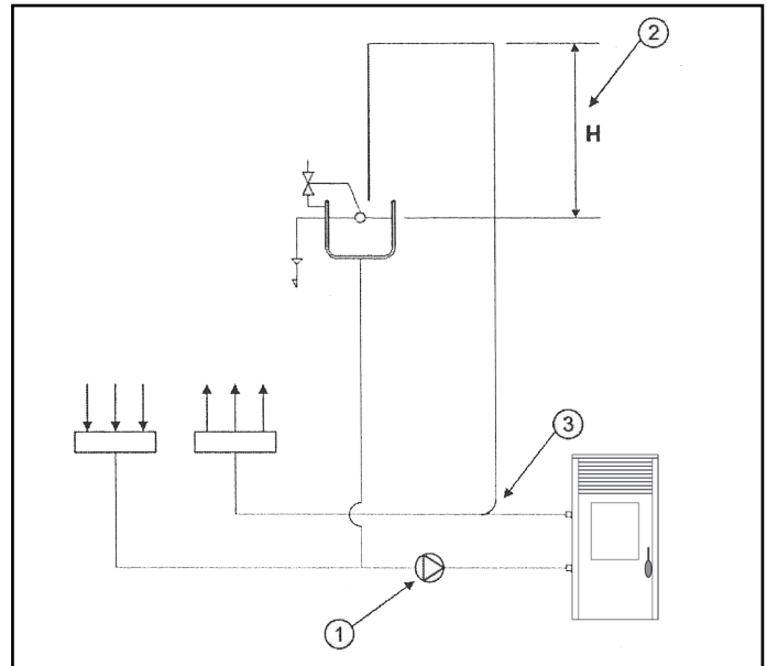
Schéma raccordement hydropoêle sans kit production eau sanitaire
