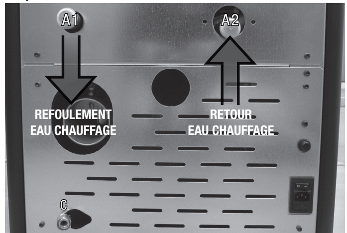
Schéma raccordement hydropoêle sans kit production eau sanitaire
