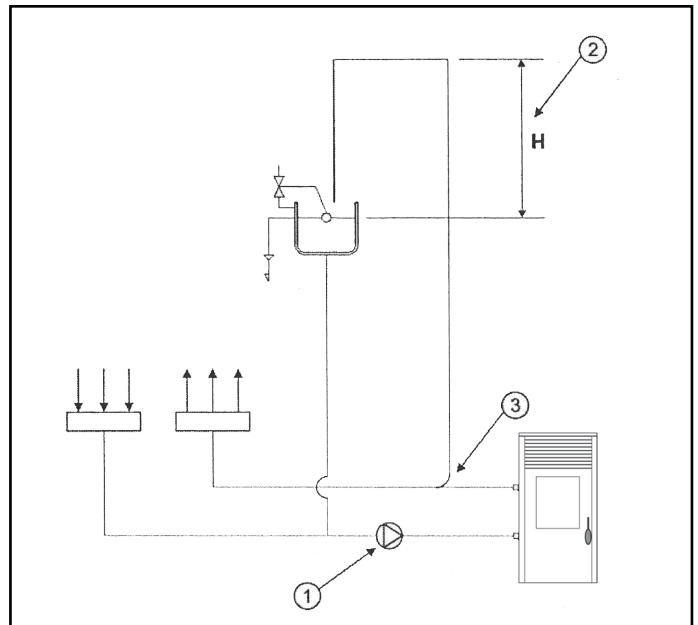
Anschlussleitung Heizofen ohne Brauchwasser-Set
