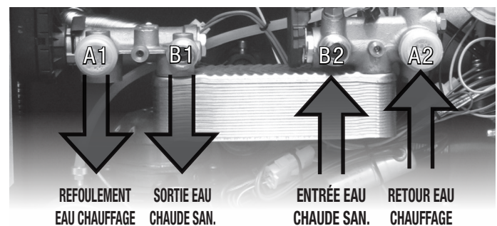
Schéma raccordement hydropoêle avec kit production eau sanitaire
