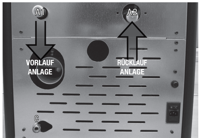
Anschlussleitung Heizofen ohne Brauchwasser-Set
