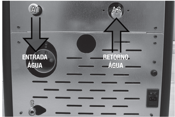
Diagrama de ligação para termo estufa sem kit de água quente sanitária
